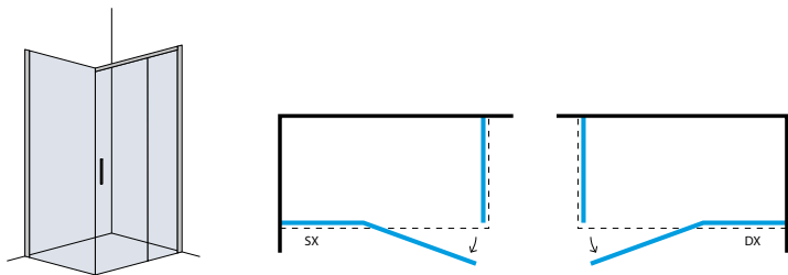
Porta battente da abbinare alla parete fissa - finitura cromo, nickel, bianco opaco, nero opaco Pivot door for fixed glass - chrome, nickel, matte white, matte black finishes
