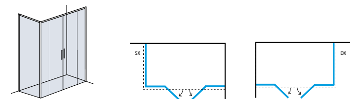
Parete fissa da abbinare alla porta doppio battente - finitura cromo, nichel, bianco opaco, nero opaco Fixed glass for double pivot door - chrome, nickel, matte white, matte black finishes
