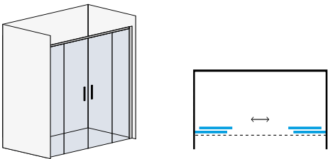
Porta doppio scorrevole - finitura cromo, nickel, bianco opaco, nero opaco Double sliding door - chrome, nickel, matte white, matte black finishes
