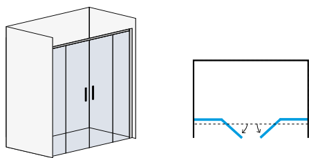
Porta doppio battente- finitura cromo, nichel, bianco opaco, nero opaco Double pivot door - chrome, nickel, matte white, matte black finishes
