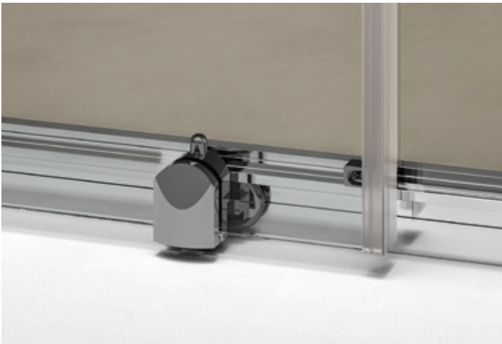
PORTA SCORREVOLE CON CHIUSURA MAGNETICA, KIT DI SCORRIMENTO A DOPPIA RUOTA COMPLETATO DA UN TASTO PER LO SGANCIO DELL'ANTA SLIDING DOOR WITH MAGNETIC LOCK DOUBLE WHEEL SLIDING KIT COMPLETED WITH A BUTTON FOR RELEASING THE DOOR
