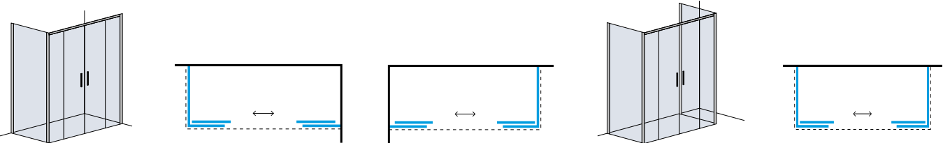
Parete fissa da abbinare alla porta doppio scorrevole - finitura nero opaco Fixed glass for double sliding door - matte black finish
