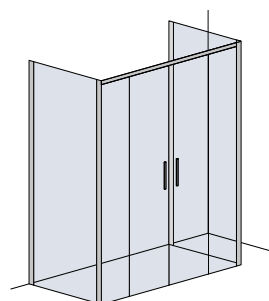
Porta doppio scorrevole + 2 Pareti fisse Double sliding door + 2 Fixed glasses
