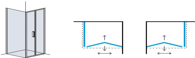
Parete fissa da abbinare alla porta pieghevole - finitura cromo Fixed glasses for bifold door - chrome finish
