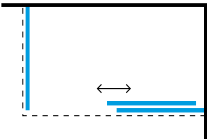
Porta doppio scorrevole + Parete fissa Double sliding door + Fixed glass
