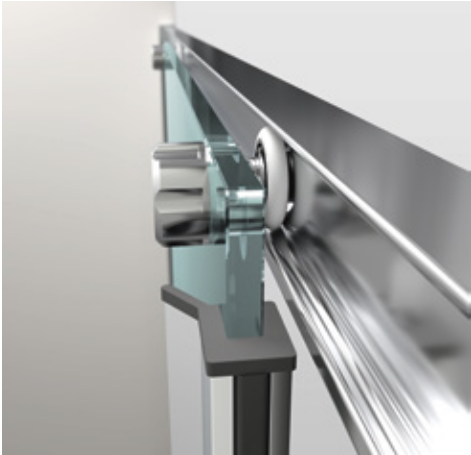
CUSCINETTI A SFERA A REGOLAZIONE ECCENTRICA ADJUSTABLE BALL BEARINGS
