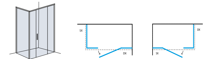
Parete fissa da abbinare alla porta battente + 2 fissi - finitura cromo, nichel, bianco opaco, nero opaco Fixed glass for pivot door + 2 fixed glasses - chrome, nickel, matte white, matte black finishes
